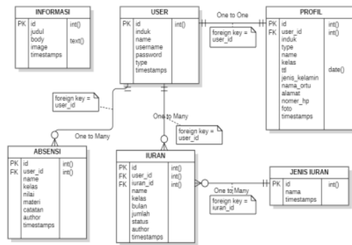
Gambar 3. ER Diagram
