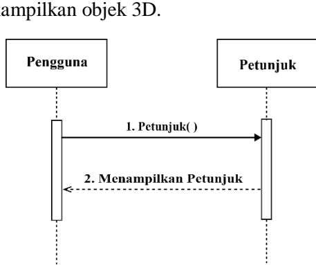
Gambar 17. Sequence Diagram Petunjuk Aplikasi
