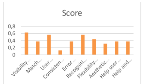
Gambar 12. Hasil Heuristic Evaluation
