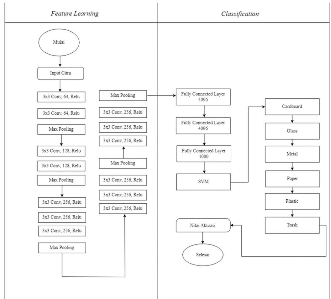
Gambar 7. Diagram Model Pelatihan Setelah Hybrid
