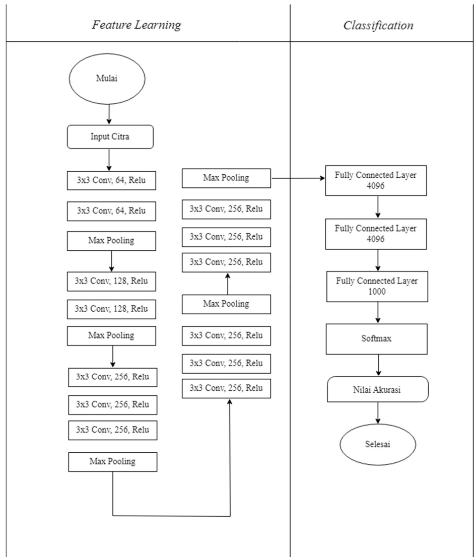
Gambar 6. Diagram Model Pelatihan Sebelum Hybrid
