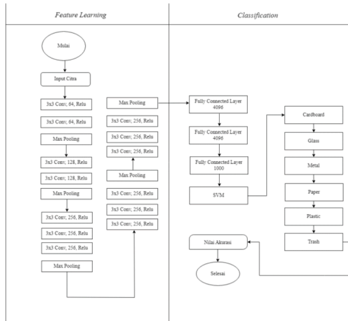
Gambar 3.9 Diagram Model Pelatihan Setelah Hybrid
