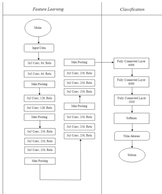
Gambar 3.8 Diagram Model Pelatihan Sebelum Hybrid
