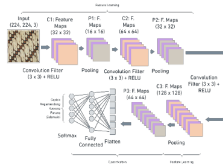
Gambar 3. Arsitektur Model CNN
