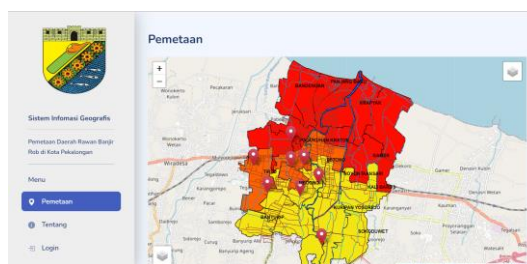
Gambar 13. Halaman Pemetaan
