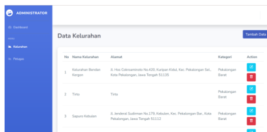
Gambar 8. Menu Kelurahan
