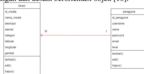
Gambar 5. Diagram Class Sistem Pemetaan Daerah Rawan Rob
