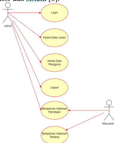
Gambar 2. Diagram Use Case Sistem Pemetaan Daerah Rawan Rob di Kota Pekalongan
