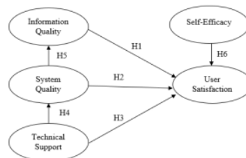
Gambar 2. Kerangka Teori
