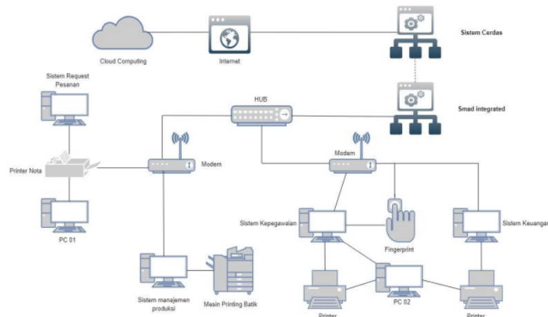
Gambar 5. Infrastruktur TI
