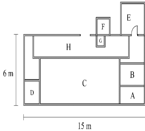
Gambar 2. Tata Letak Awal
