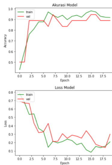
Gambar 6. Visualisasi nilai akurasi dan loss model dengan menggunakan hyperparameter
