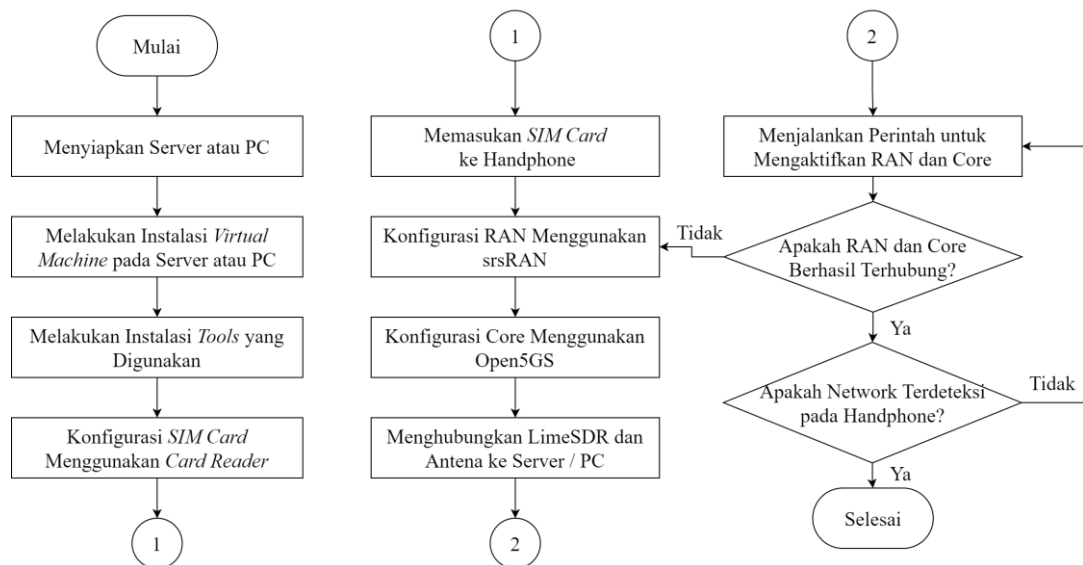
Gambar 4. Alur Pembuatan Jaringan Open RAN 4G pada Server / PC
