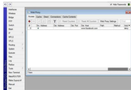
Gambar 11. Web Proxy
