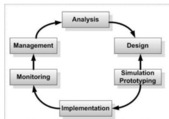
Gambar 1. Rancangan Analisis
