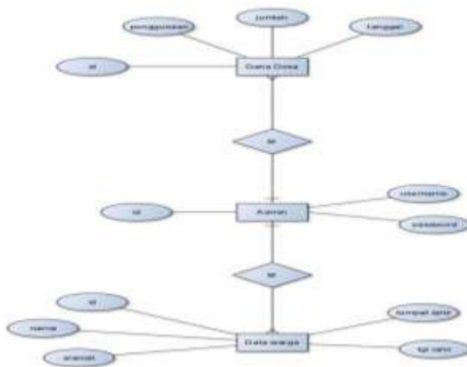
Fig.4. ERD
