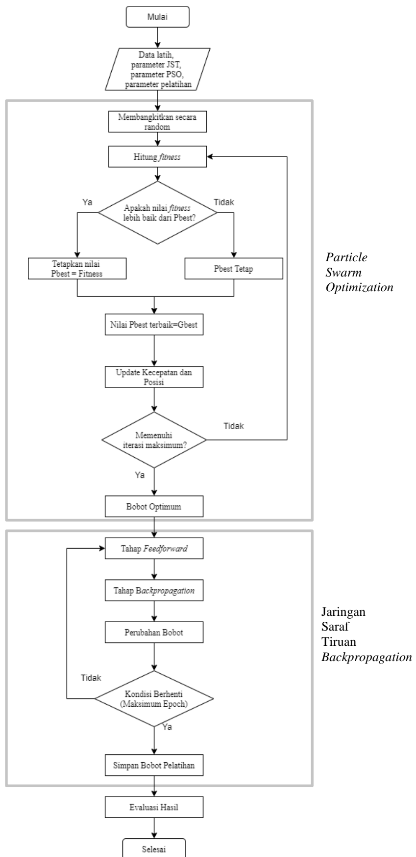
Gambar 2. Tahap Pelatihan Prediksi Pasien Penyakit Ginjal Kronis Hibrid JST-PSO
