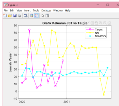
Gambar 5. Perbandingan Nilai Prediksi dan Target Proses Pelatihan
