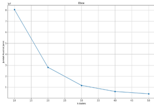
Gambar 3.5 Pencarian k dengan elbow
