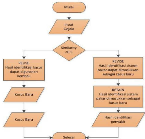
Gambar 3. Flowchart Sistem Pakar dengan Proses CBR
