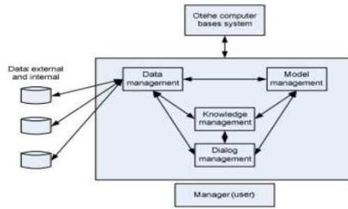
Gambar 1. Komponen-komponen Sistem Pendukung Keputusan
