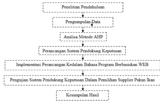
Gambar 3. Kerangka Kerja
