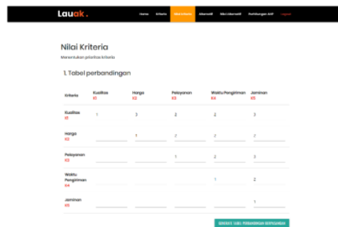
Gambar 5. Matriks Skala Perbandingan berpasangan
