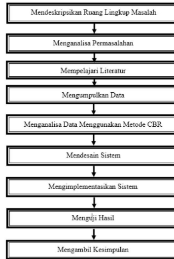
Gambar 1. Metodologi Penelitian
