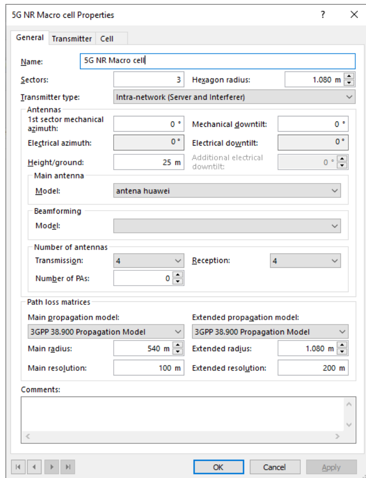
Gambar 3.13 5G NR Macro cell properties di atoll 3.4
