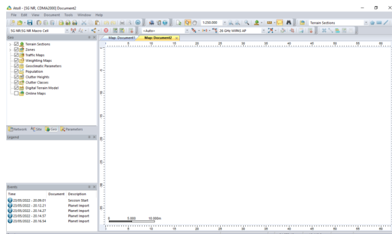
Gambar 3.3 Aplikasi atoll 3.4
