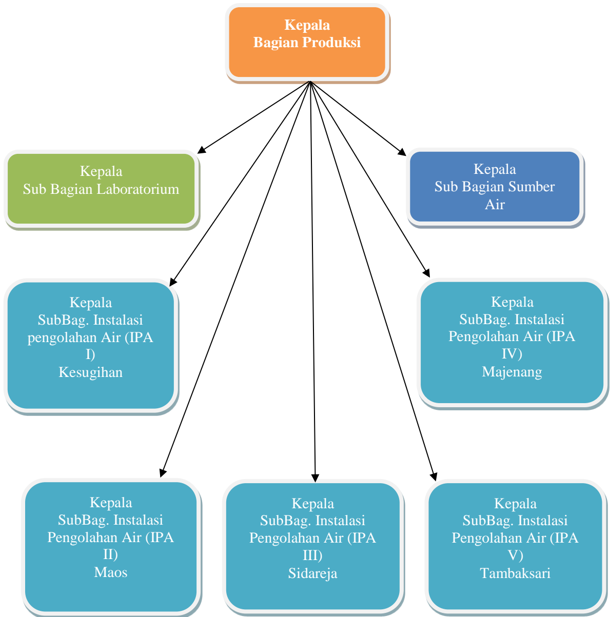
Gambar 2.1 Struktur Organisasi
