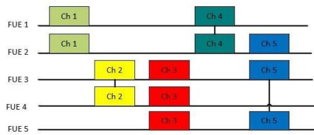
Gambar 3. 4 Skema Penggunaan Channel pada 5 User [16]
