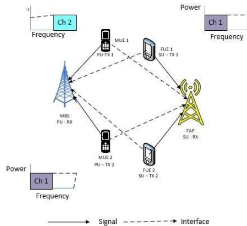
Gambar 3. 2 Model User dan Channel pada Jaringan Heterogen [14]
